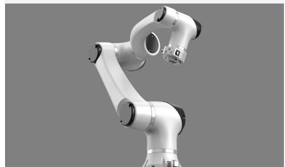
Kollaborative Roboter, sog. "Cobots", von Han's Robot. Die Traglast der Roboter variiert von 3 kg bis 18 kg. Die Wiederholgenauigkeit liegt bei \pm 0,02\text{mm} in der hochpräzisen Ausführung. Diese Cobots zeichnen sich durch technische Überlegenheit und kompromisslose Sicherheit aus.
