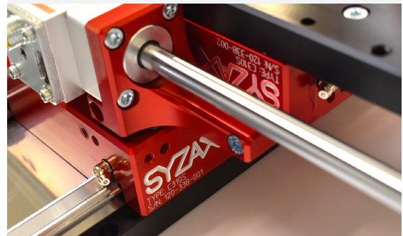
Lineartechnik "Syzax" von Opus S.A. für standardisierte und konfigurierbare modulare Linearmotoren, geeignet für hochpräzise Handhabungsmodule mit einer Genauigkeit von \pm 3\mu\text{m} in kompakter Bauweise.
